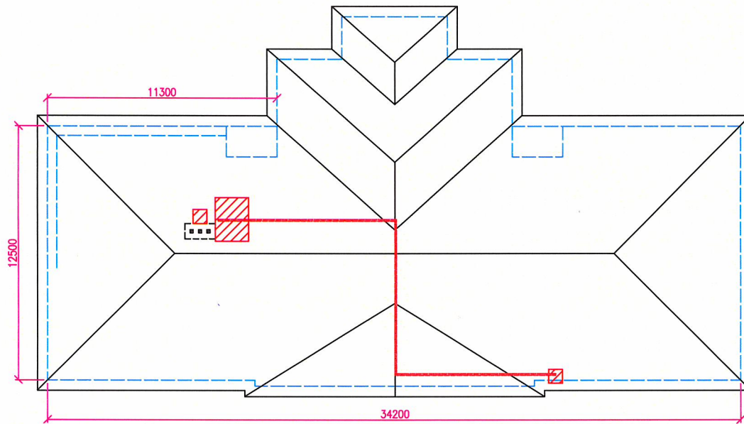
PŮDORYS
